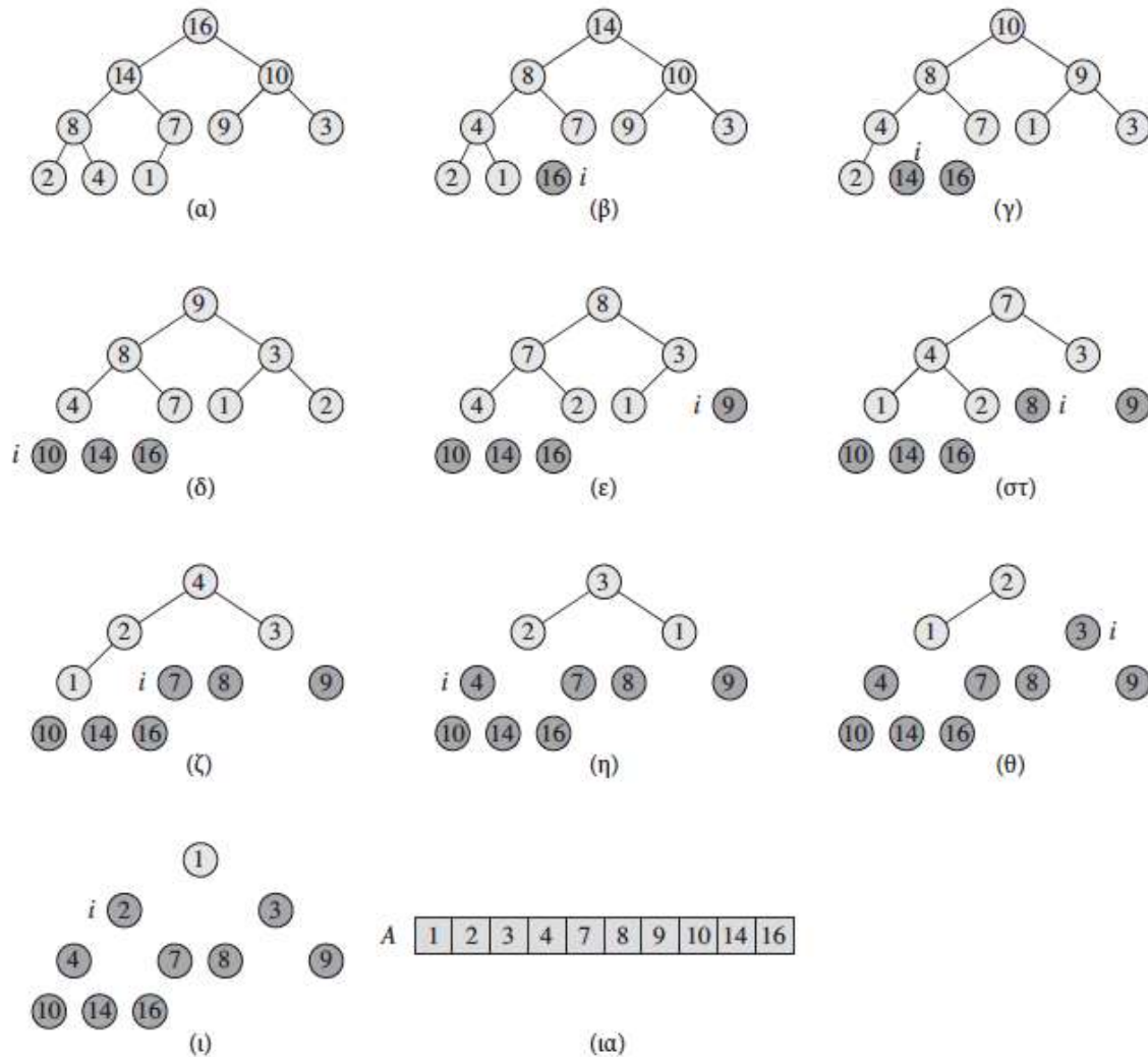
Σχήμα 6.4 Η λειτουργία της ΤΑΞΙΝΟΜΗΣΗΣ ΣΩΡΟΥ. (α) Η δομή δεδομένων του σωρού μεγίστου αμέσως μετά την κατασκευή της μέσω της ΚΑΤΑΣΚΕΥΗΣ ΣΩΡΟΥ ΜΕΓΙΣΤΟΥ στη γραμμή 1. (β)–(i) Οι διαδοχικοί σωροί μεγίστου αμέσως μετά την κάθε κλήση της ΑΠΟΚΑΤΑΣΤΑΣΗΣ ΣΩΡΟΥ ΜΕΓΙΣΤΟΥ στη γραμμή 5. Στο κάθε σχήμα υποδεικνύεται επίσης η τιμή του i τη δεδομένη χρονική στιγμή. Μόνο οι ελαφρά σκιασμένοι κόμβοι εξακολουθούν να ανήκουν στον σωρό. (ia) Η τελική ταξινομημένη συστοιχία A .
