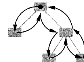
An Euler tour.
