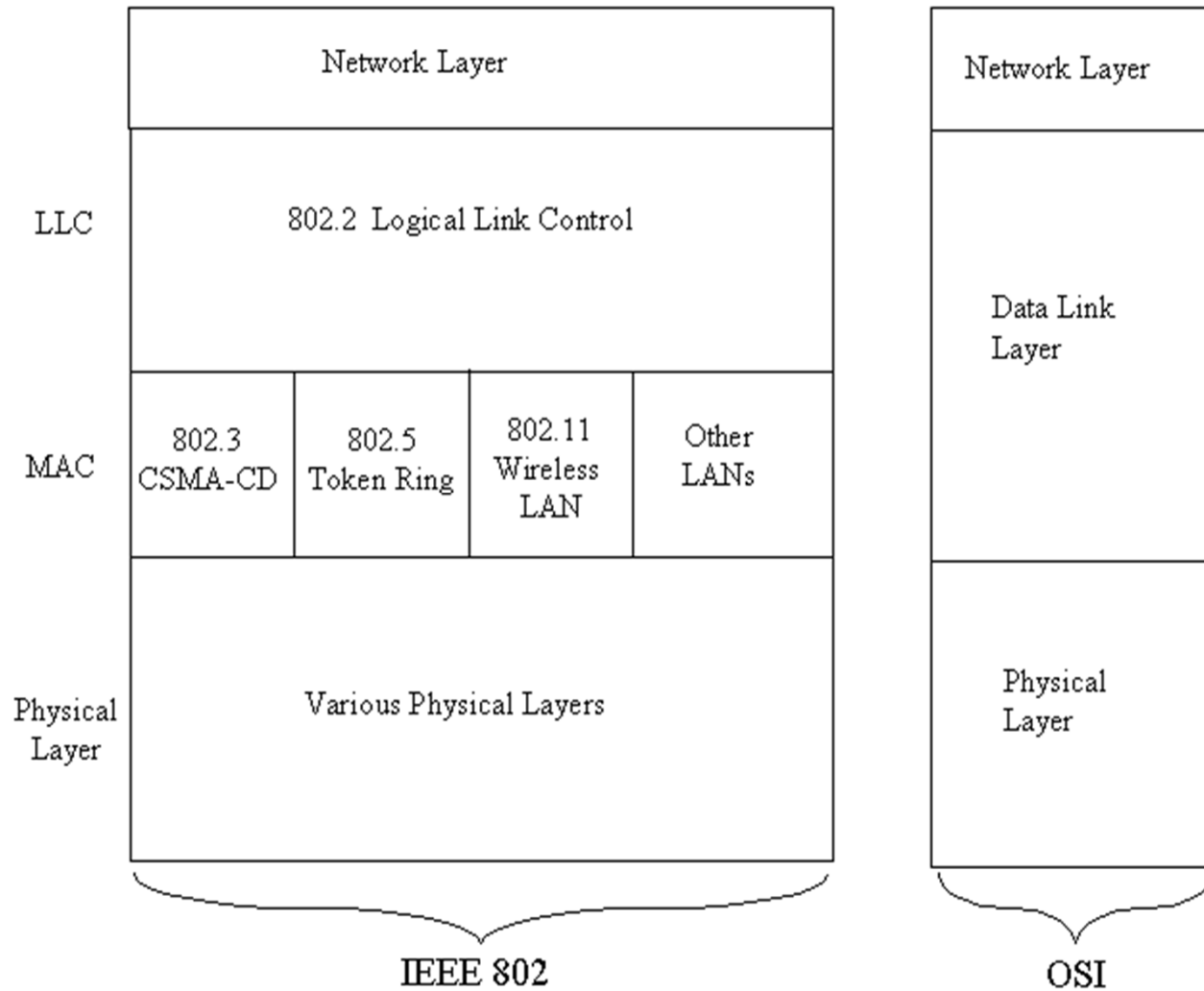
Αντιπαράθεση του IEEE 802 με το μοντέλο OSI
