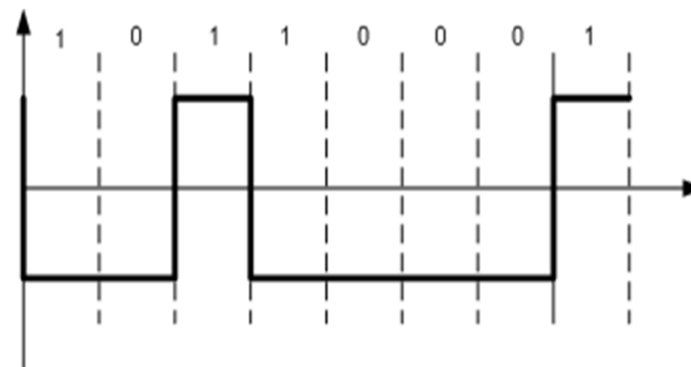
Μέθοδος κωδικοποίησης NRZ-I
