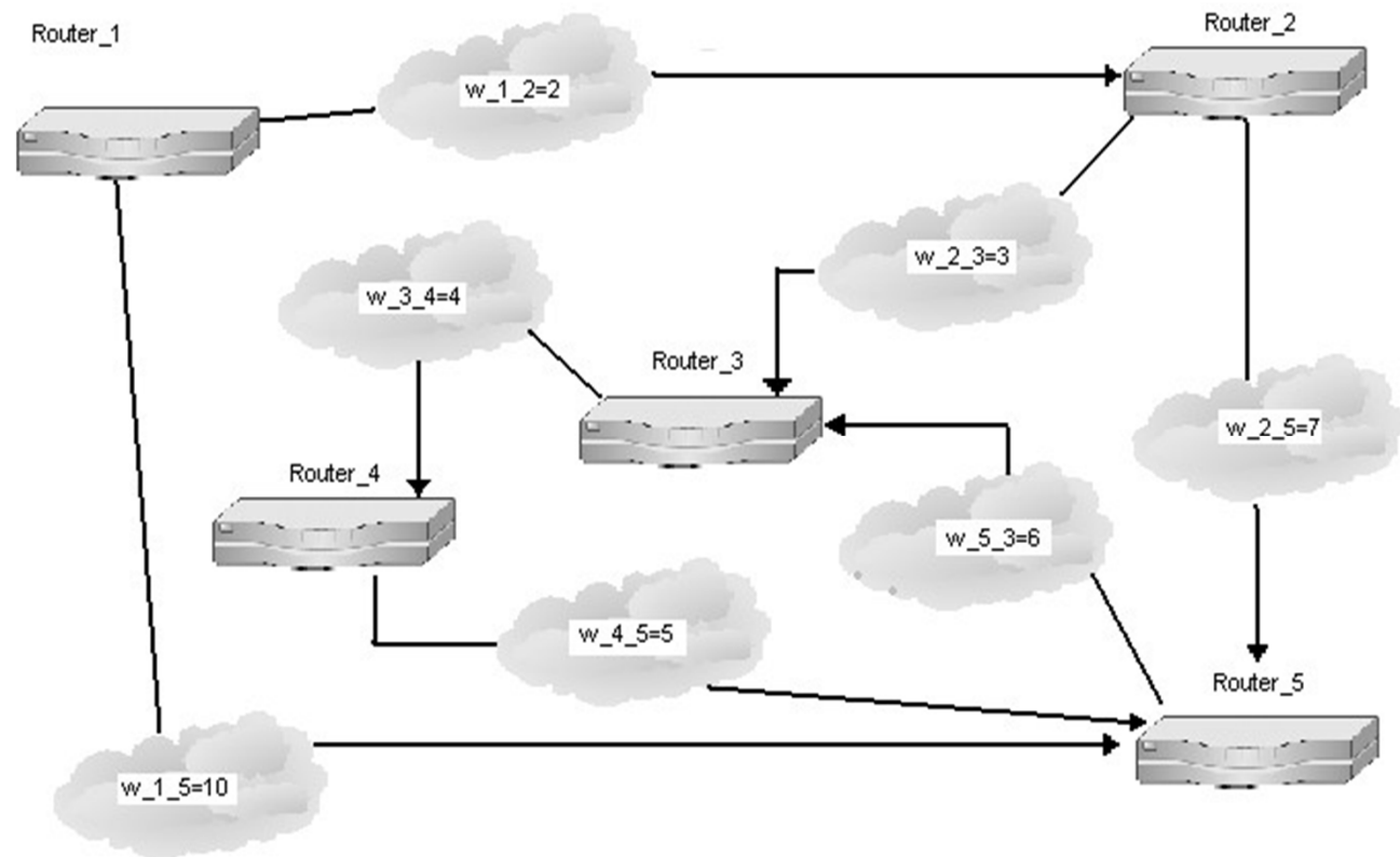
Παράδειγμα αλγόριθμου Dijkstra
